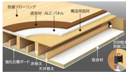
▲界床断面イメージ図
